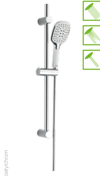
ZESTAW NATRYSKOWY NA DRAŻKU wymiar słuchawki: 241x105 mm długość drążka: 700 mm
