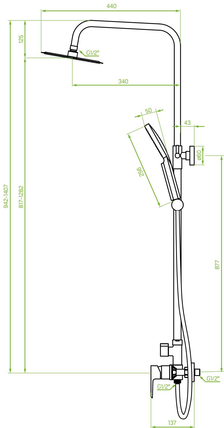
LAVEO - LARGO PAH x00B 1:7 (mm)
