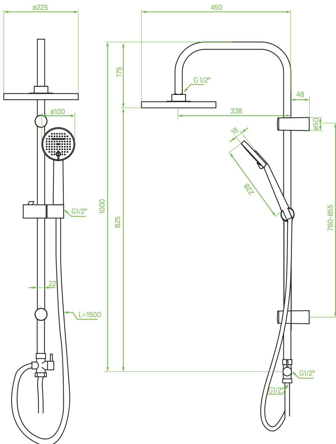
LAVEO - LESTE PLL 200X 1:7 (mm)
